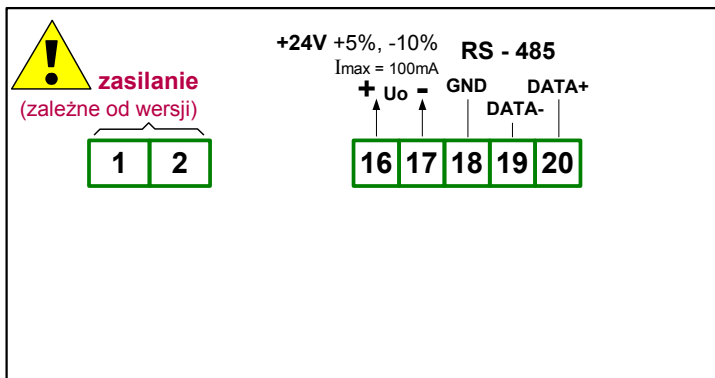
Rys. 4.5. Opis wyprowadzeń
