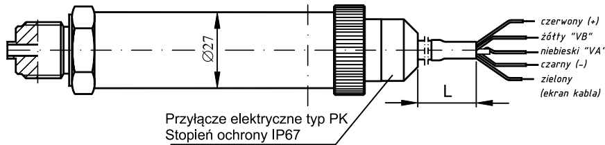
Rys. I.1. Przyłącze typu PK.
