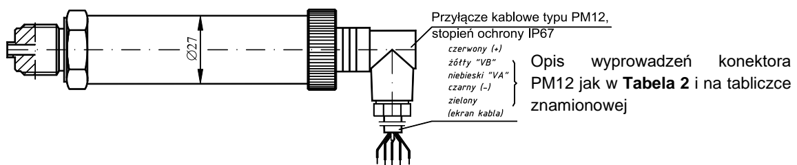
Rys. I.4. Przyłącze typu PM12.
