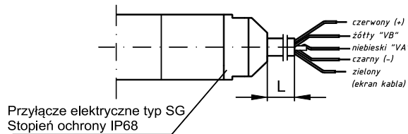
Rys. I.3. Przyłącze typu SG.
