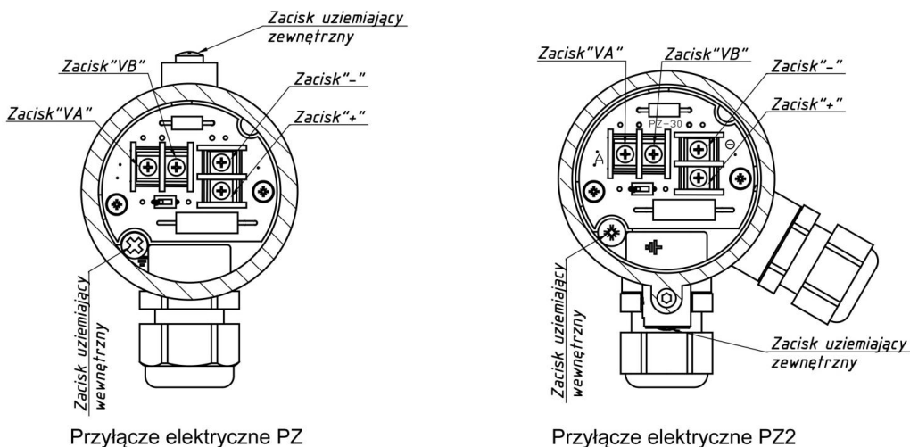
Rys. I. 5. Przyłącze typu PZ i PZ2.
