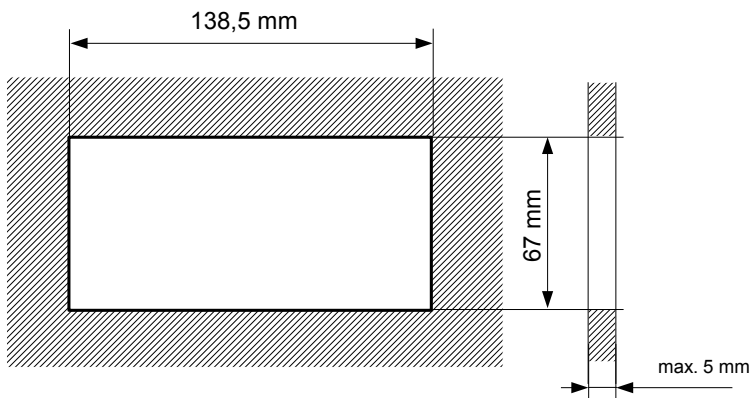
Rys. 4.1. Wymiary montażowe: a) zalecane, b) dopuszczalne
