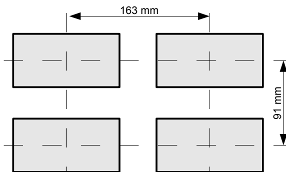
Rys. 4.3. Montaż wielu urządzeń
