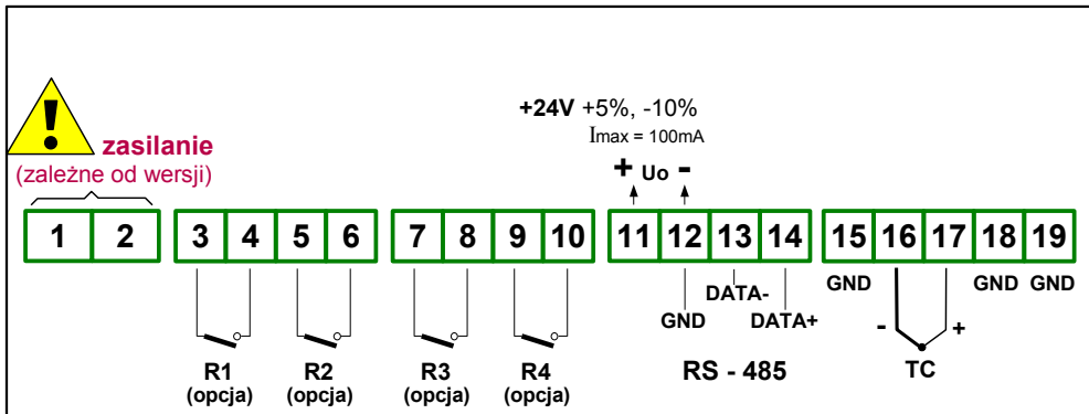
Rys. 4.5. Opis wyprowadzeń dla wersji z wyjściami przekaźnikowymi, bez wyjścia prądowego
