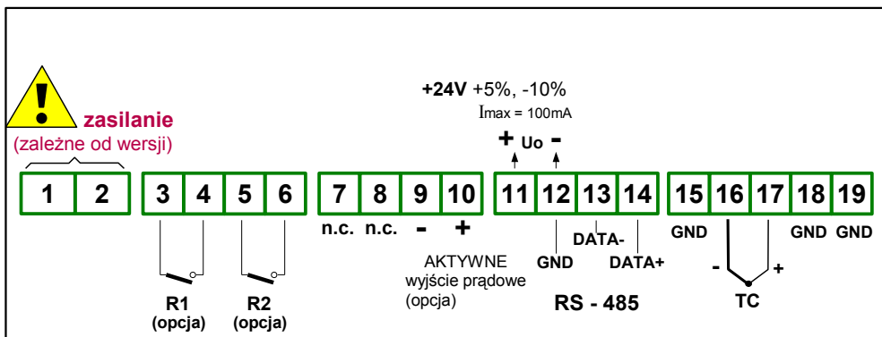
Rys. 4.6. Opis wyprowadzeń dla wersji z wyjściami przekaźnikowymi oraz aktywnym wyjściem prądowym
