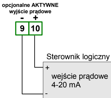
Rys. 4.11. Przykład podłączenia wyjścia prądowego (tylko dla urządzeń posiadających wyjście prądowe)
