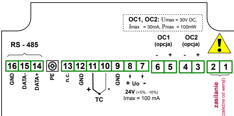
Rys. 4.5. Opis wyprowadzeń dla wersji z wyjściami OC
