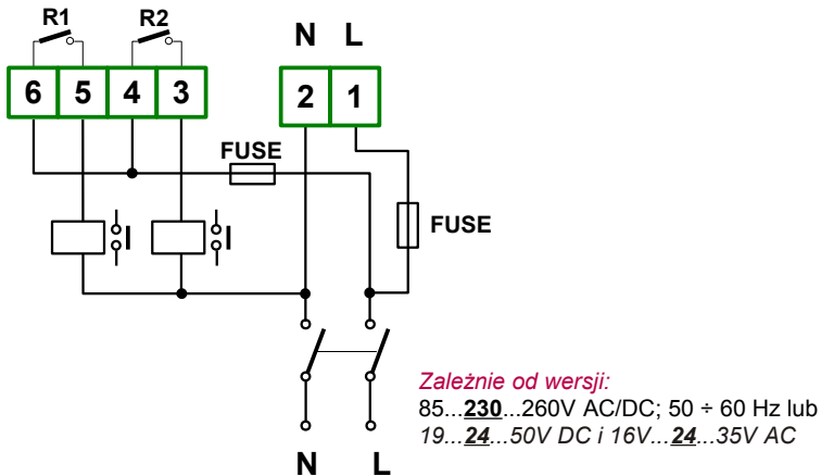
Rys. 4.8. Podłączenie przekaźników sterujących obciążeniami
