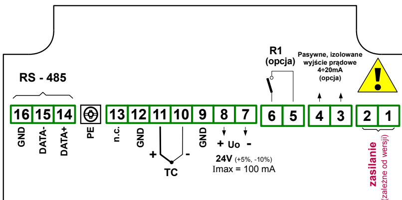
Rys. 4.6. Opis wyprowadzeń dla wersji z wyjściem przekaźnikowym oraz prądowym
