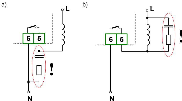
Rys. 4.9. Przykłady równoległego podłączenia obwodu tłumiącego: a) do styków przekaźnika; b) do obciążenia indukcyjnego
