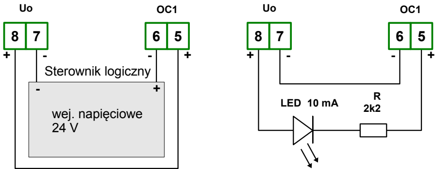
Rys. 4.10. Przykładowe podłączenia wyjścia typu OC
