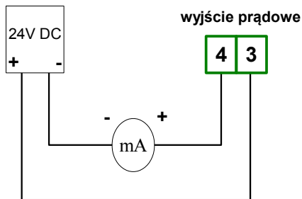
Rys. 4.12. Przykładowe podłączenie wyjścia prądowego używając zewnętrznego źródła zasilania
