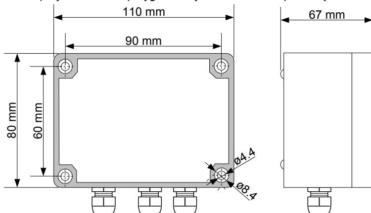
Rys. 4.1. Wymiary montażowe
