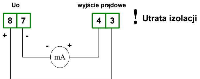
Rys. 4.11. Przykładowe podłączenie wyjścia prądowego używając wewnętrznego źródła zasilania
