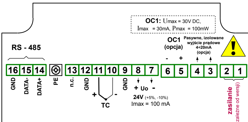
Rys. 4.7. Opis wyprowadzeń dla wersji z wyjściem OC oraz prądowym
