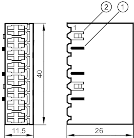
Rysunek przedstawia obudowę złącza z zamkniętą pokrywą Widok od strony styków
