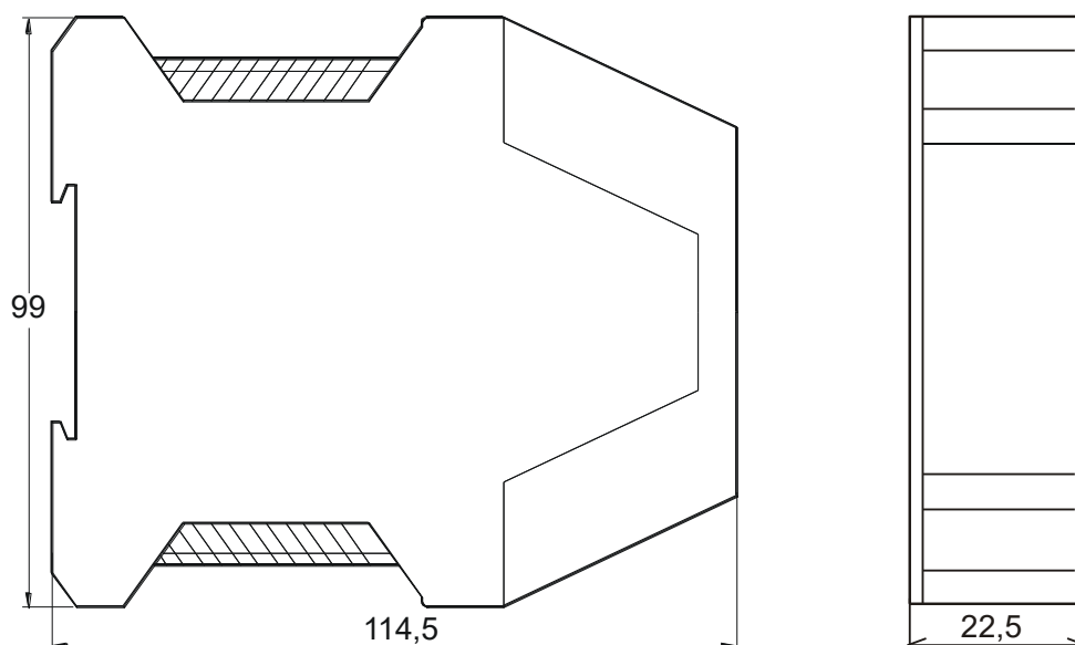
Szkic obudowy.
